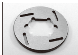
SPブレーキディスク SP Brake Disk No.IFW122 ★1890 研磨済みディスク Polished High Strength
