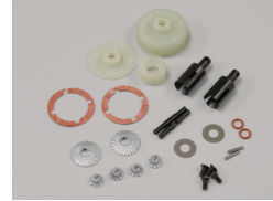
UMW604B ギヤデフセット Gear Diff. Set
