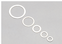
96641/96643/96647 シムセット Shim Set ※96641 3x5mm(0.1/0.2/0.3mm)各10入 (0.1/0.2/0.3mm)10pcs ※96643 5x7mm(0.1/0.2/0.3mm)各10入 (0.1/0.2/0.3mm)10pcs ※96647 10x12mm(0.1厚/0.2厚)各4入 (0.1/0.2)4pcs
