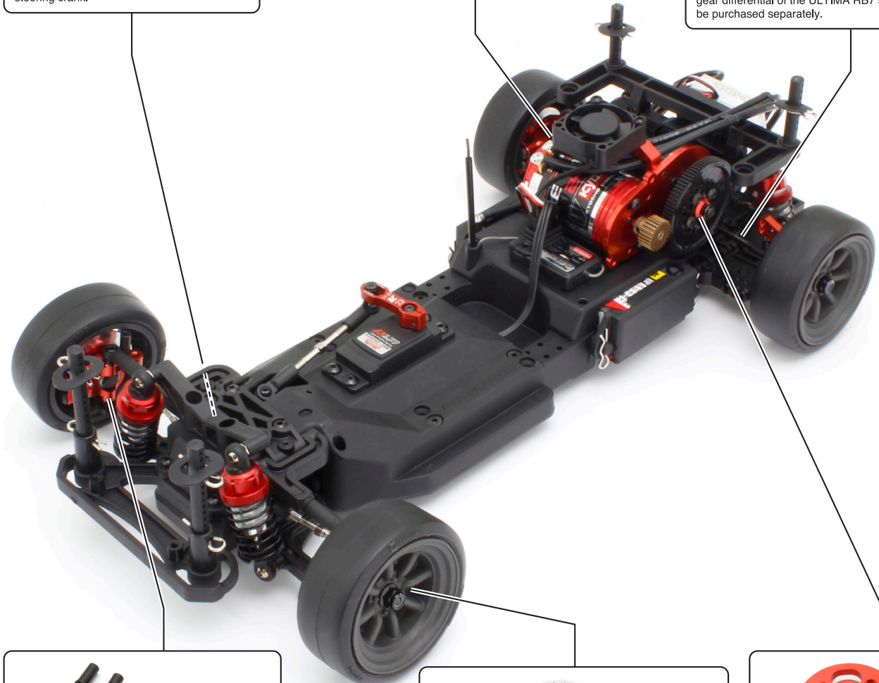
No.FAW303 ステアリングクランクピン(FZD2/2入) Steering Clank Pin (FZD2/2pcs) ステアリングクランクの剛性と精度を向上。 Improved rigidity and precision of the steering crank.
